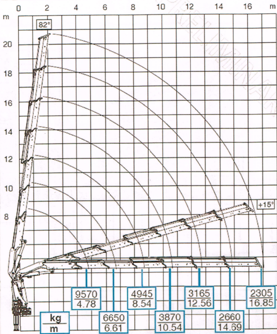
Hefcapaciteiten 525 ROOFCRANE
